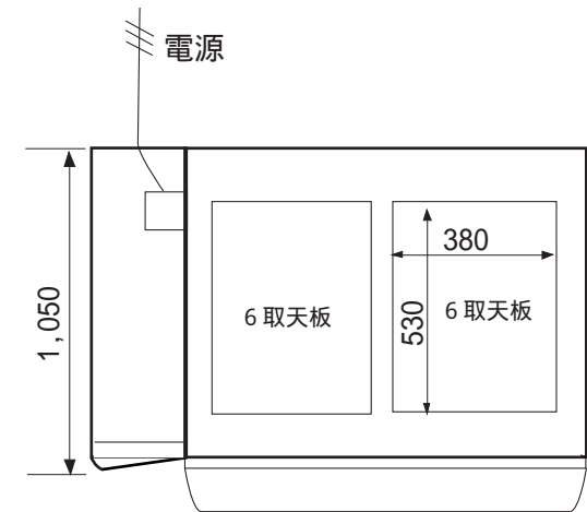
MFB-6 承認図 左BOX (アジャスト 90mm)
